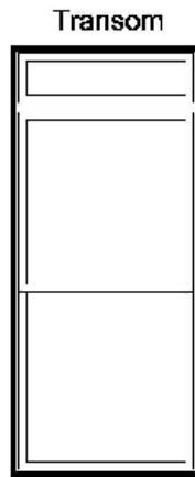
3060 36" X 84"
